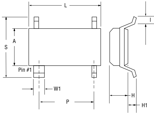
SOT - 143
