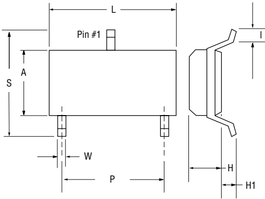
SOT - 23
